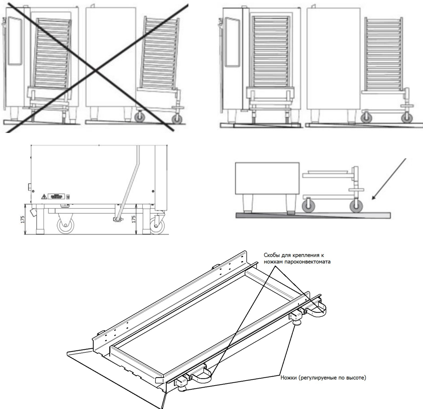
Подставка ПТП-20
